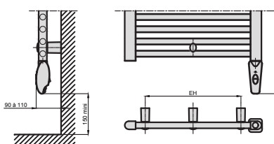
VERSION ELECTRIQUE A LIAISON RF
