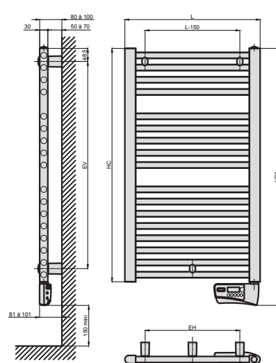
VERSION MIXTE RACCORDEMENT CENTRAL 50 MM A LIAISON RF
