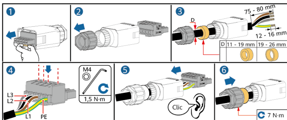
Figure 5-6 Câble à quatre conducteurs (L1, L2, L3 et PE)
