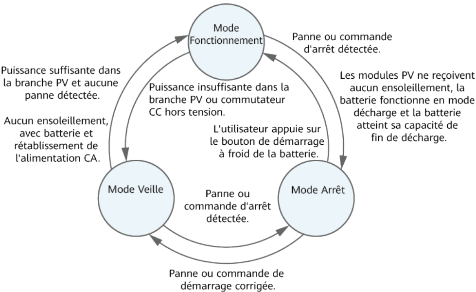
Figure 2-11 Modes de fonctionnement
