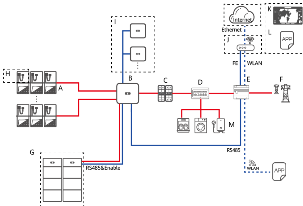
Figure 2-3 Mise en réseau du SmartAssistant (les composants dans les encadrés en pointillé sont facultatifs)
