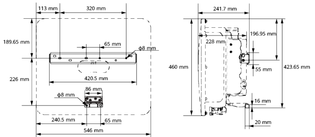
Figure 4-1 Dimensions de l'onduleur et du support de montage
