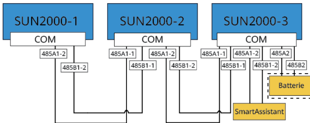
Figure 5-19 Mise en réseau SmartAssistant (les composants dans les encadrés en pointillé sont facultatifs)
