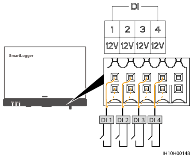
Figure 5-39 Connexions des câbles (mise en réseau du SmartLogger)
