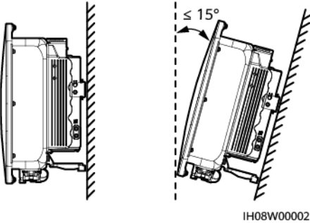
Figure 4-5 Angle d'installation
