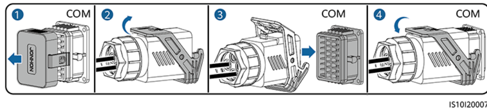
Figure 5-22 Fixation du connecteur du câble de signal
