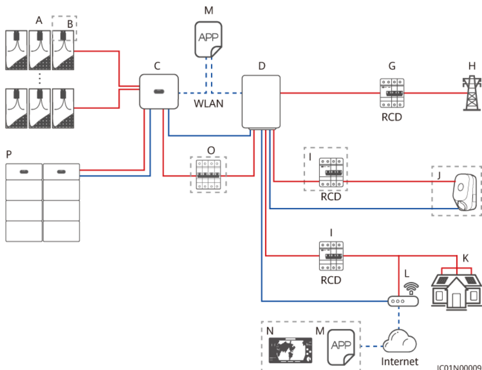
Figure 2-4 Mise en réseau avec toutes les charges connectées au SmartGuard (les composants dans les encadrés en pointillé sont facultatifs)
