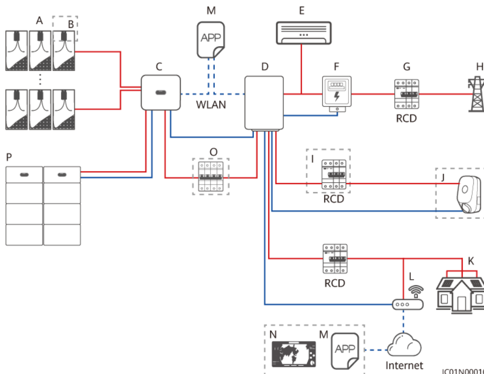
Figure 2-5 Mise en réseau avec certaines charges connectées au SmartGuard (les composants dans les encadrés en pointillé sont facultatifs)
