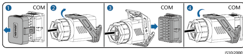
Figure 5-41 Fixation du connecteur du câble de signal
