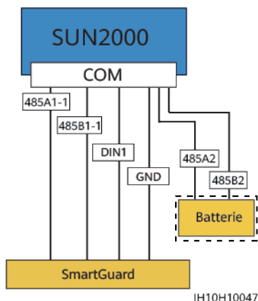
Figure 5-20 Mise en réseau SmartGuard (les composants dans les encadrés en pointillé sont facultatifs)
