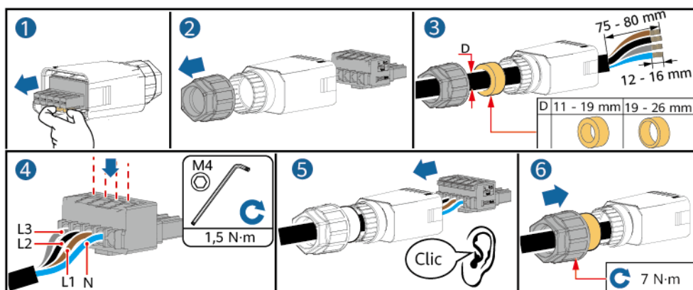
Figure 5-7 Câble à quatre conducteurs (L1, L2, L3 et N)
