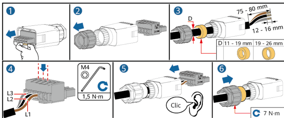
Figure 5-5 Câble à trois conducteurs (L1, L2 et L3)
