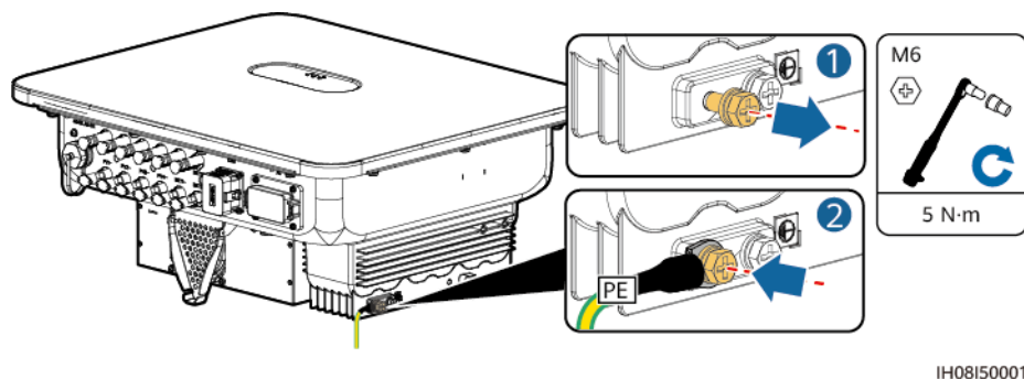
Figure 5-3 Connexion du câble PE
