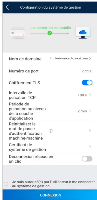
Figure D-1 Déconnexion du réseau en un clic (exemple pour l'utilisateur de l'installateur)
