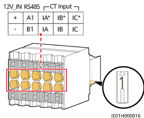
Figure 5-5 Connecteur 10 broches
