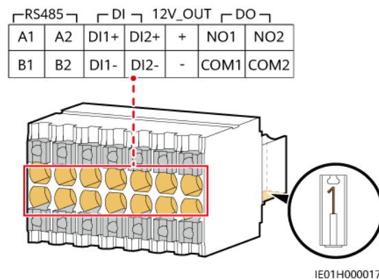
Figure 5-9 Connecteur 14 broches
