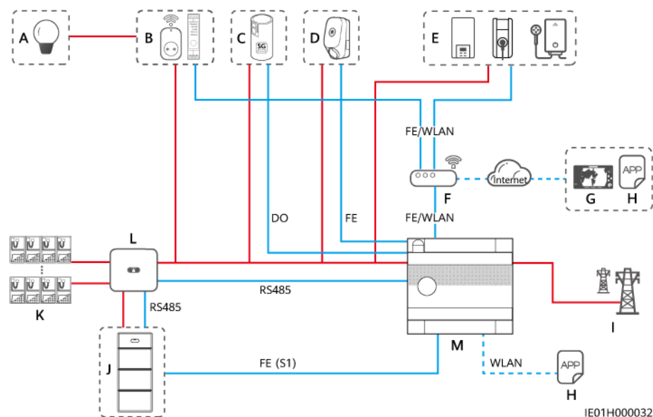
Figure 2-2 Diagramme de mise en réseau (en utilisant l'EMMA-A02 comme exemple)
