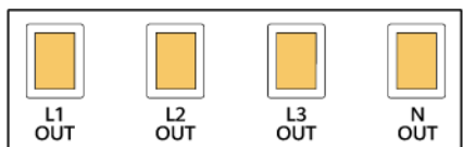
Figure 5-4 Ports du câble d'alimentation de sortie CA
